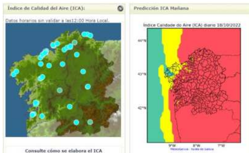
Figura 8.14 Estaciones ICA e índice de calidad de aire a diario. Fuente: www.meteogalicia.gal
