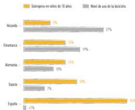
Figura 1.1: Relación entre sobrepeso infantil y el uso de la bicicleta en países europeos
