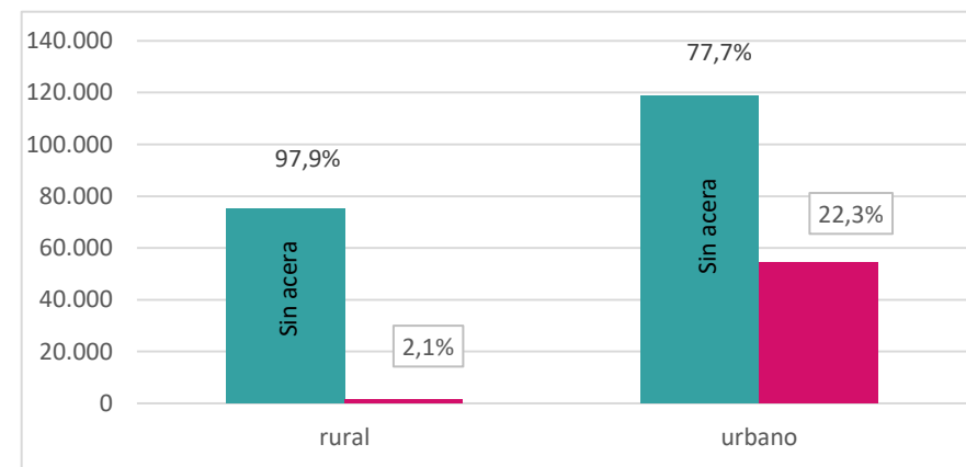
Figura 7.1 Porcentaje de calles con y sin aceras según ámbito rural o urbano
