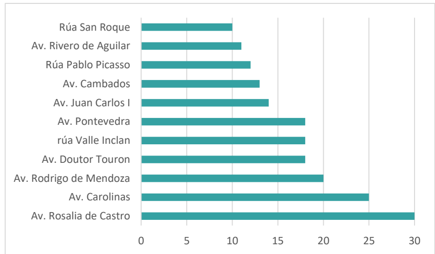
Figura 8.13 Número de accidentes por calle en 2021. Fuente: Policía local
