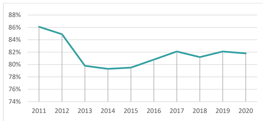
Figura 4.7 Autosuficiencia en empleo (porcentaje de personas que trabajan en el mismo municipio). Fuente: IGE
