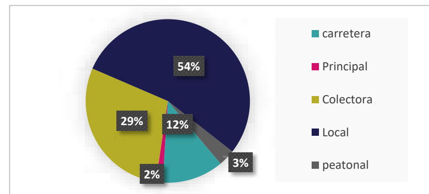
Figura 7.2 Reparto de las tipologías de viales en el municipio.
