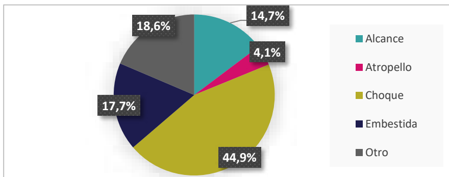
Figura 8.12 Tipo de accidentes de tráfico en 2021. Fuente: Policía local
